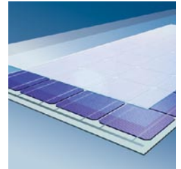
Modulaufbau: speziell gehärtetes eisenarmes Glas / lichtdurchlässige Ethyl-Vinyl-Acetat (EVA)-Folie / Solarzellen / EVA / Rückseitenfolie
